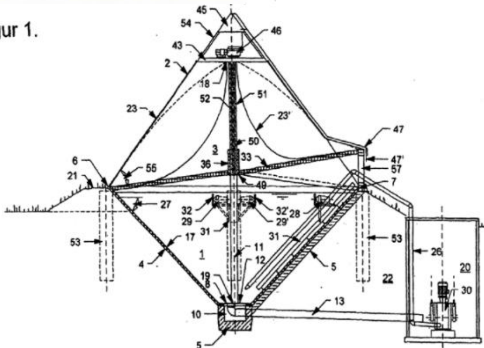
SCHNITT A-A
